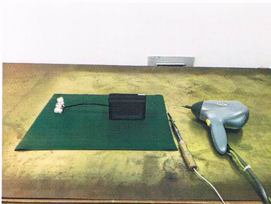
静电放电抗扰度-模式 1
