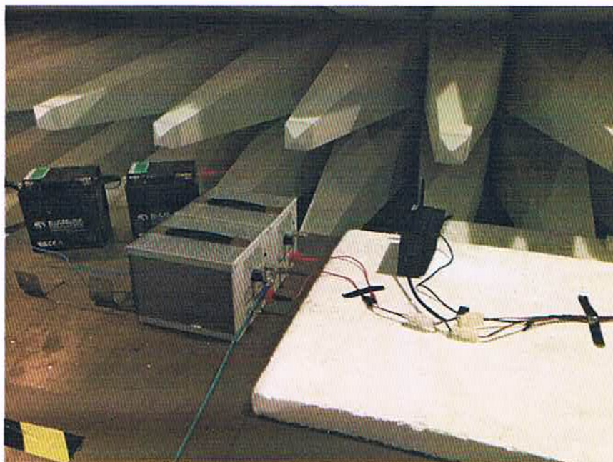
传导发射 (电压法)
