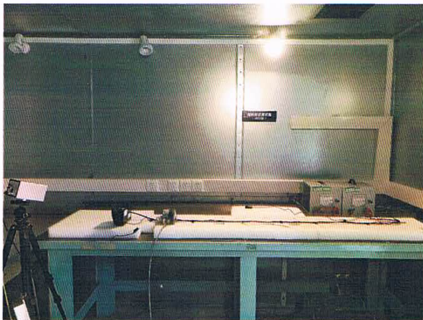
大电流注入抗扰度 (BCI 法)
